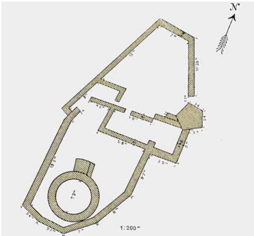
Tloris utvrde Nečven
